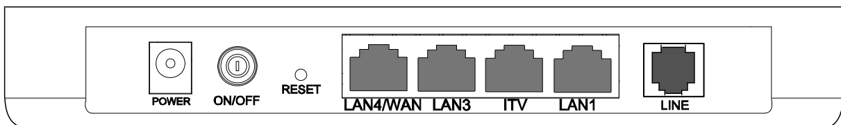
图 2 TD-89402 后面板示意图
